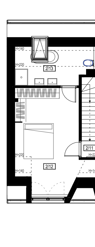
PODDASZE
