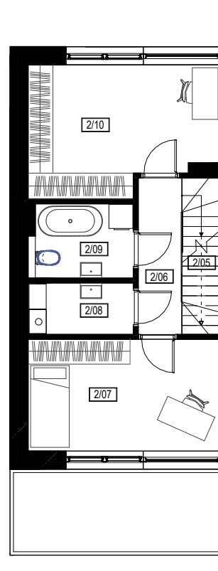
I PIĘTRO
