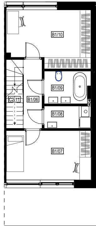
I PIĘTRO
