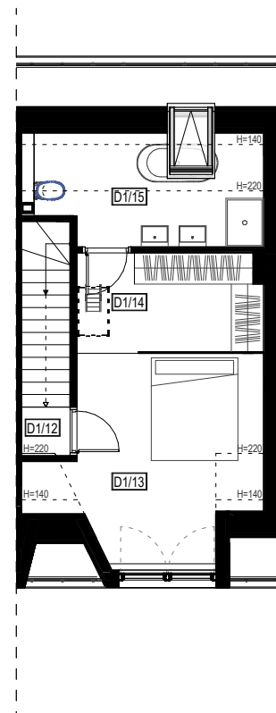
PODDASZE
