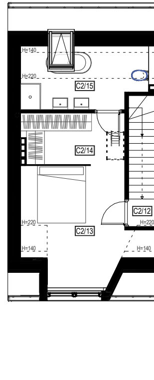
PODDASZE
