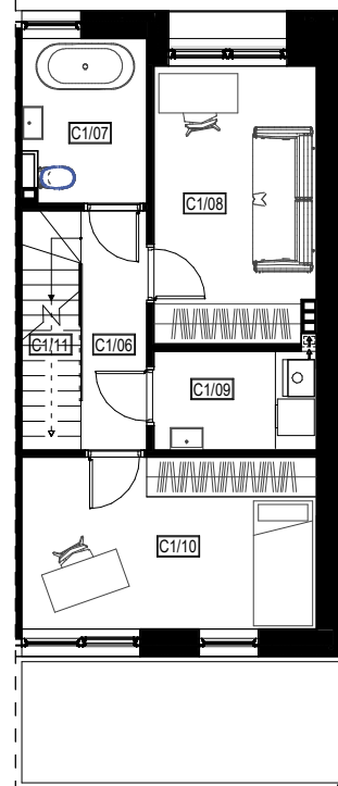
I PIĘTRO
